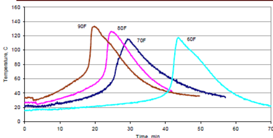
不同温度下 10g MA422 的标准放热曲线 5
