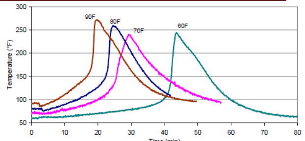
不同温度下 10g MA422 的标准放热曲线 5
